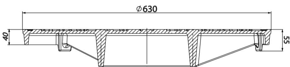
Frame art. 630F KBT D400
