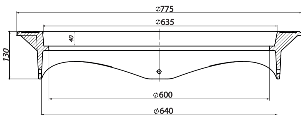
Frame art. 630F KBT D400
